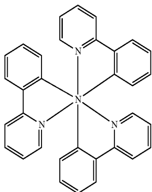
[Ir(ppy) 3 ]
